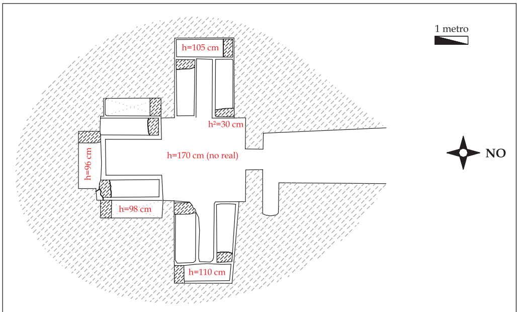
FIGURA 99. Planta del hipogeo QM G/7. Tipo 3
