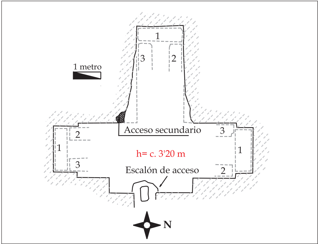
FIGURA 53. Planta del hipogeo QM C2/13. Tipo 3
