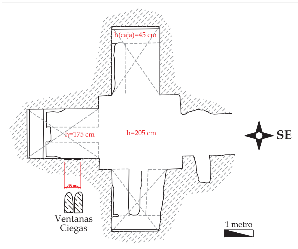
FIGURA 47. Planta del hipogeo QM C2/10. Tipo 3
