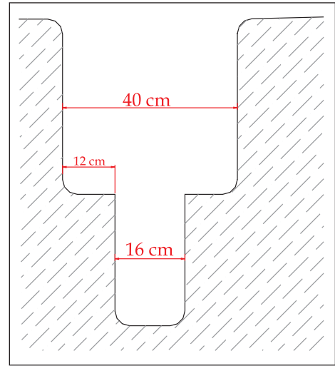
FIGURA 107. Sección del canal
