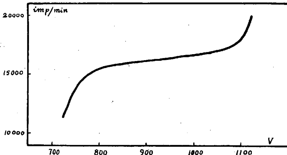
Figura 1.—Curva característica del tubo G-M utilizado con el equipo de contaje «Philips»
