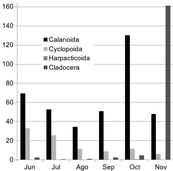
Figura 3. Abundancia total mensual (ind/L) de los grupos taxonómicos más representativos del macrozooplancton registrados en la laguna Sauce Grande entre junio y noviembre de 2010.
