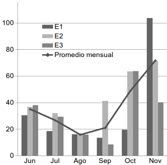
Figura 2. Abundancia total mensual (ind/L) de macrozooplancton por estación de muestreo (E1, E2, E3) y promedio mensual durante el período de estudio en la Laguna Sauce Grande.
