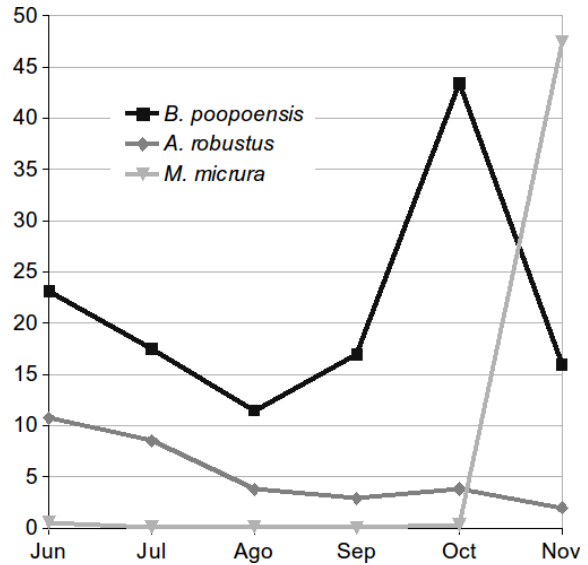
Figura 4. Abundancia promedio mensual (ind/L) de los principales taxa de macrozooplancton hallados en la laguna Sauce Grande entre junio y noviembre de 2010.
