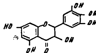
miricetina
