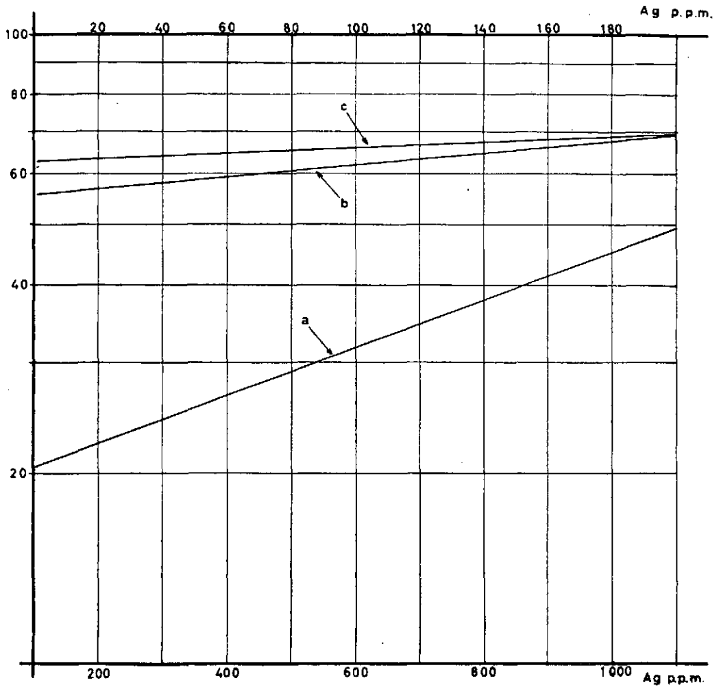
CURVA PATRON PARA DETERMINACION COLORIMETRICA DE PLATA
