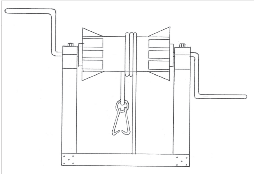
Dibujo del torno con la maroma y los ganchos.
