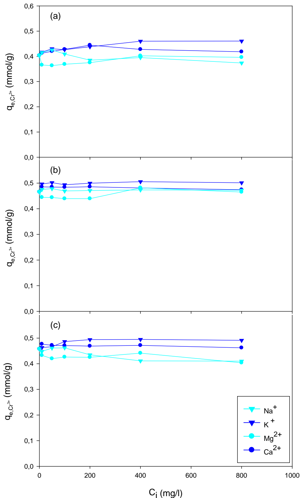
Figura V.30. Cromo adsorbido por unidad de masa de sólido adsorbente frente a la concentración de Na + , K + , Mg 2+ y Ca 2+ , para: (a) P-H 2 O (b) P-NaOH y (c) P-HCl. M_{sólido} = 0,2 g; V_{disolución} = 50 ml; pH=5,0, t_{contacto} = 48 horas.
