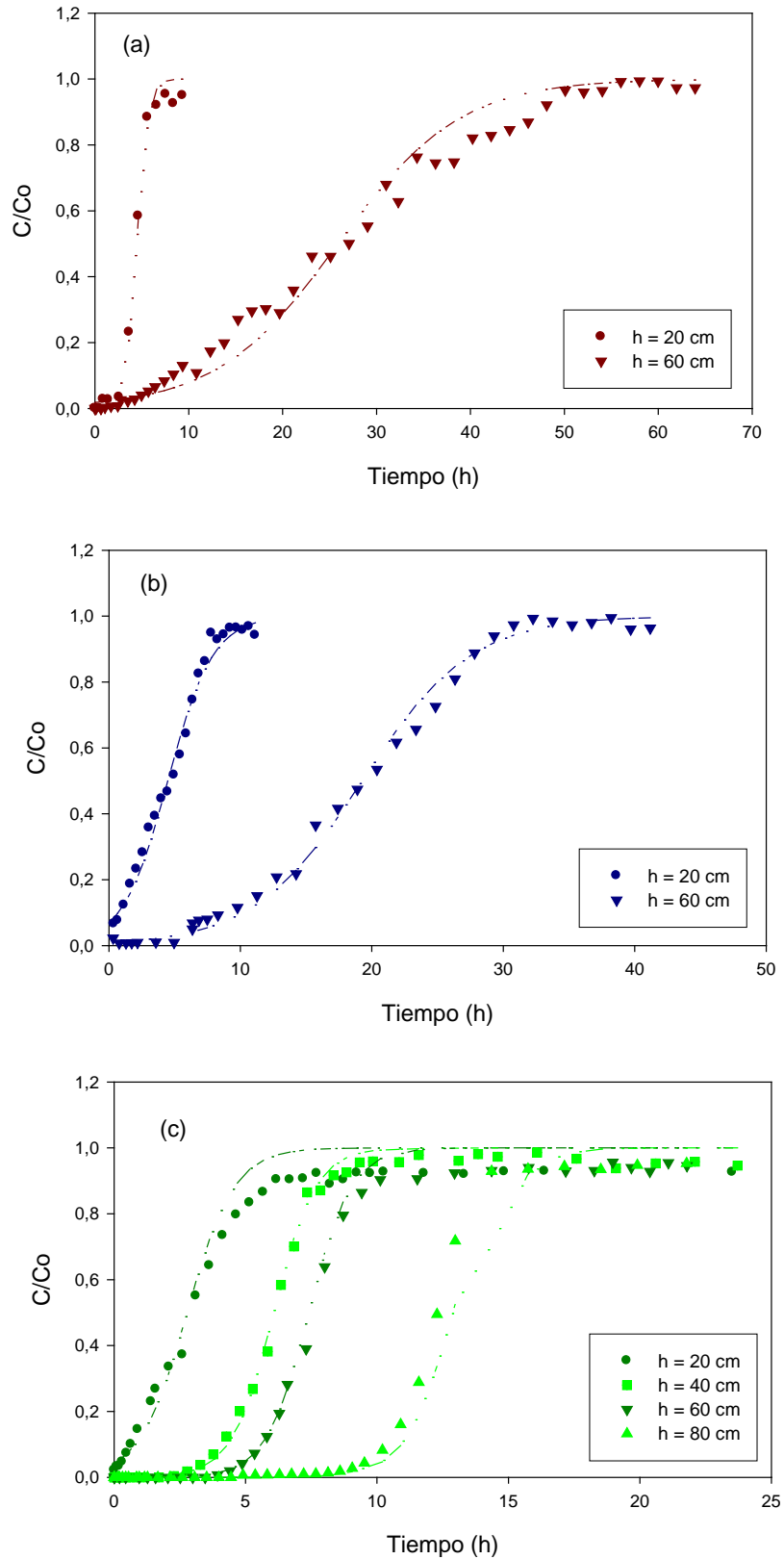
Figura VIII.6. Influencia de la altura de lecho. Mejores ajustes al modelo BDST. a) \text{Cd}^{2+} , b) \text{Zn}^{2+} y c) \text{Cr}^{3+} .
