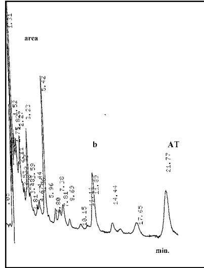
Figura 2.- Cromatograma de una muestra de huevo + \beta -tocopherol (b) + acetato de \alpha -tocopherol (AT).
