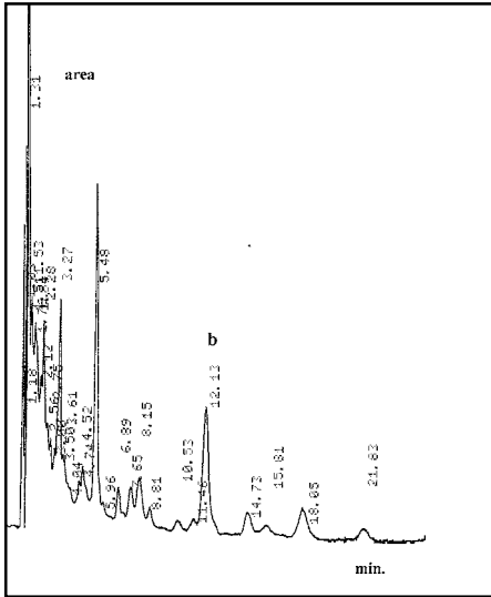
Figura 1.- Cromatograma de una muestra de huevo + \beta -tocopherol (b).
