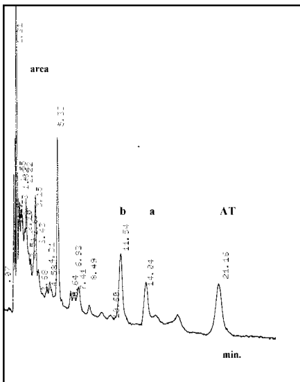
Figura 3.- Cromatograma de una muestra de huevo + \beta -tocopherol (b) + acetato (AT) de \alpha -tocopherol + \alpha -tocopherol.
