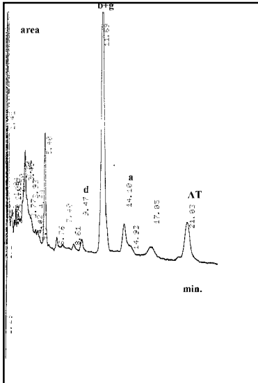
Figura 5.- Cromatograma de una muestra de huevo + \beta -tocopherol + acetato (AT) de \alpha -tocopherol + \alpha -tocopherol + \gamma -tocopherol + \delta -tocopherol.
