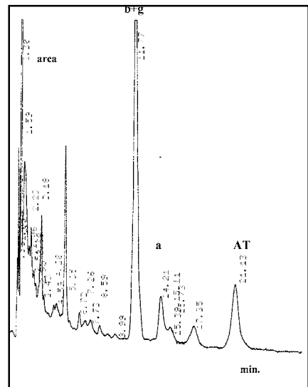
Figura 4.- Cromatograma de una muestra de huevo + \beta -tocopherol + acetato (AT) de \alpha -tocopherol + \alpha -tocopherol + \gamma -tocopherol.
