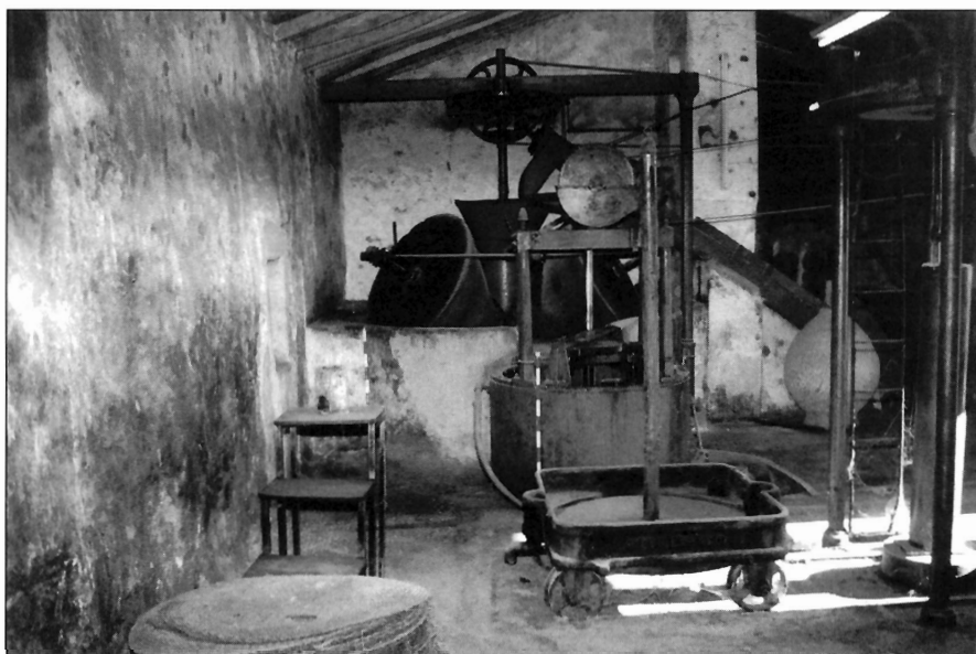
Foto 8: Vista general de la muela (8 y 9), batidora (10), prensa hidráulica (13), vagoneta y capachos (16).
