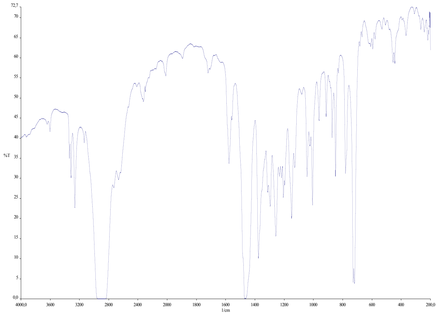
IR spectrum of 1b-Br (Nujol, cm -1 )
