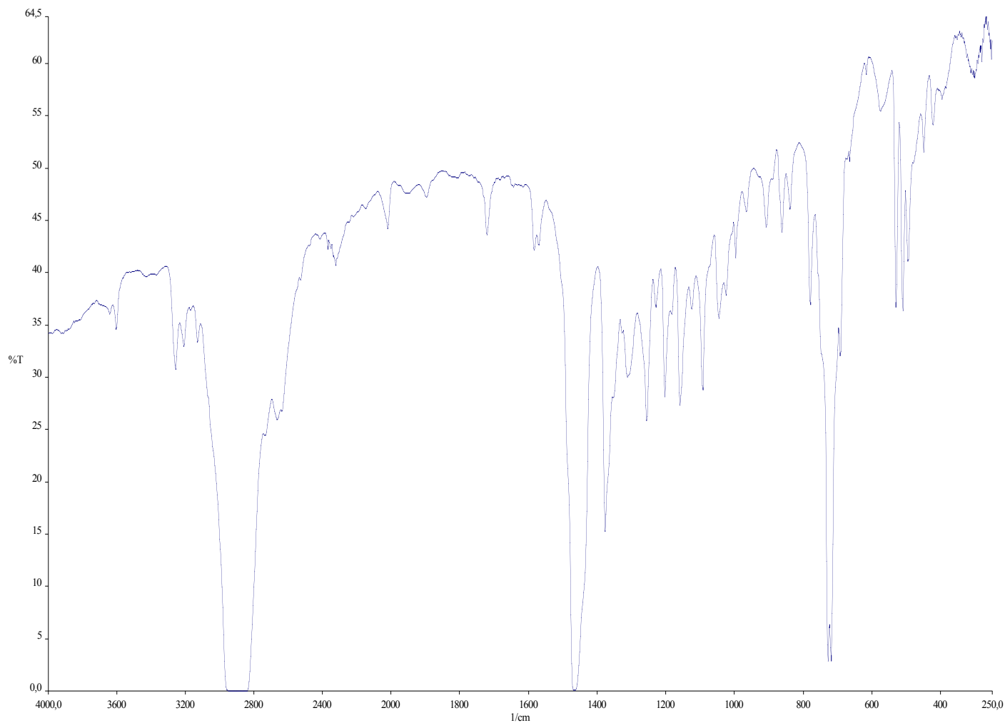
IR spectrum of 3b-Br (Nujol, cm -1 )
