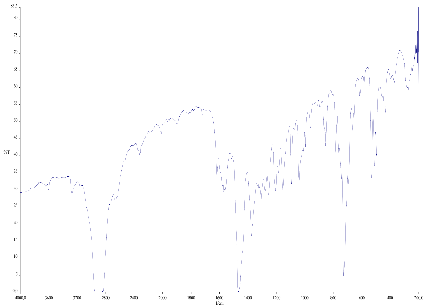
IR spectrum of 3b-OAc (Nujol, cm -1 )
