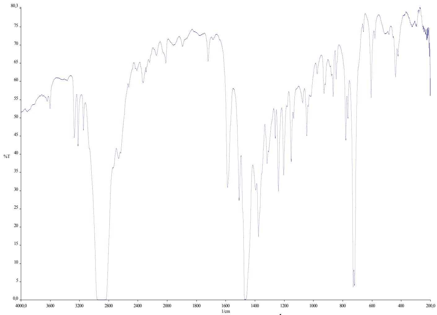
IR spectrum of 2b (Nujol, cm -1 )
