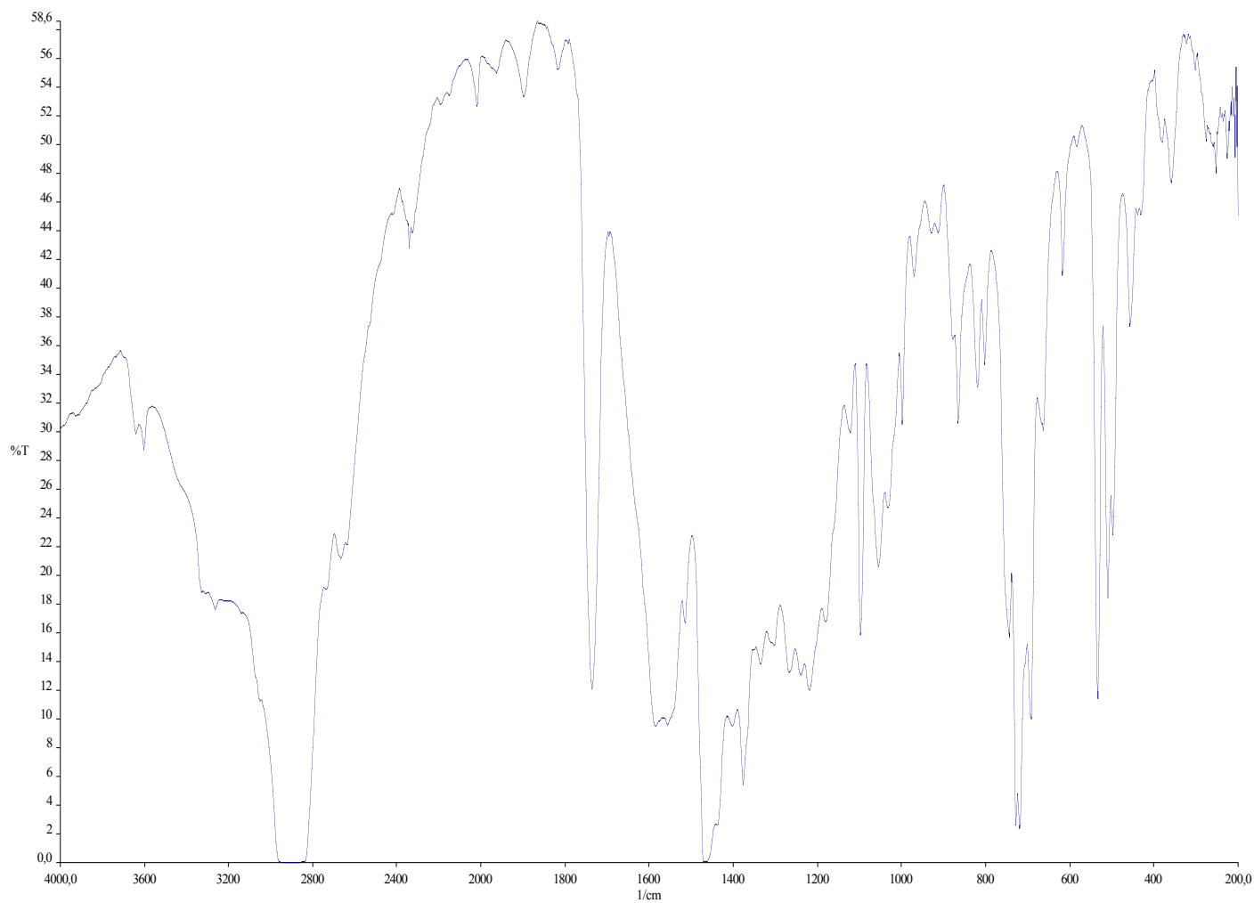
IR spectrum of 3a-OAc (Nujol, cm -1 )
