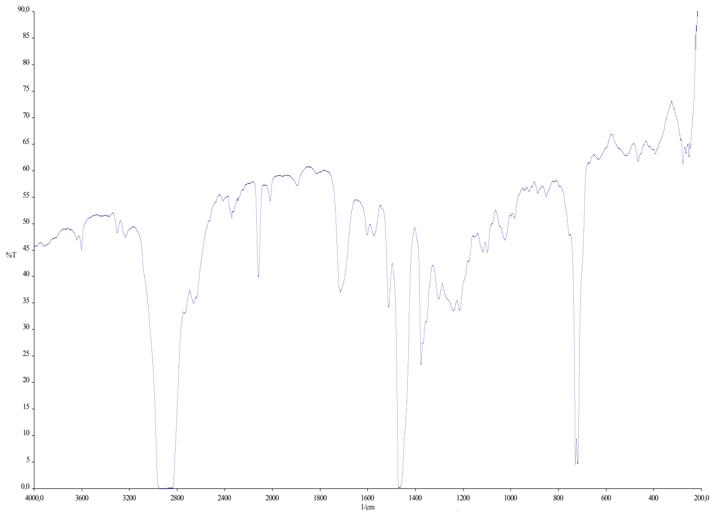
IR spectrum of 4a (Nujol, cm -1 )
