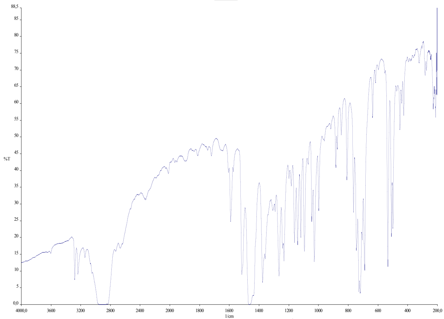
IR spectrum of 7b-Br (Nujol, cm -1 )
