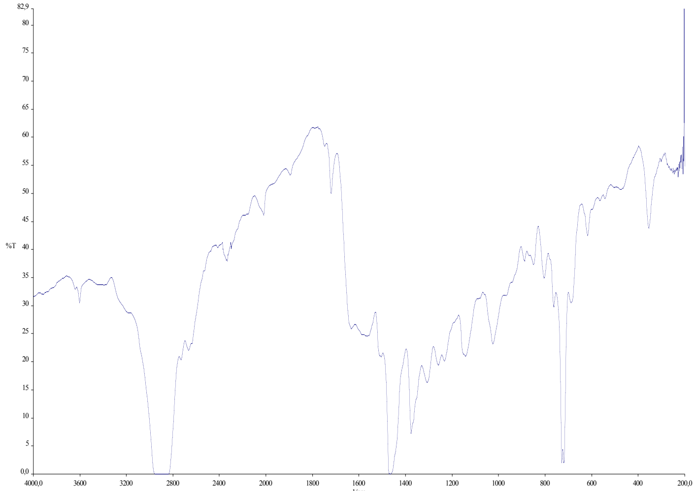
IR spectrum of 8b (Nujol, cm -1 )
