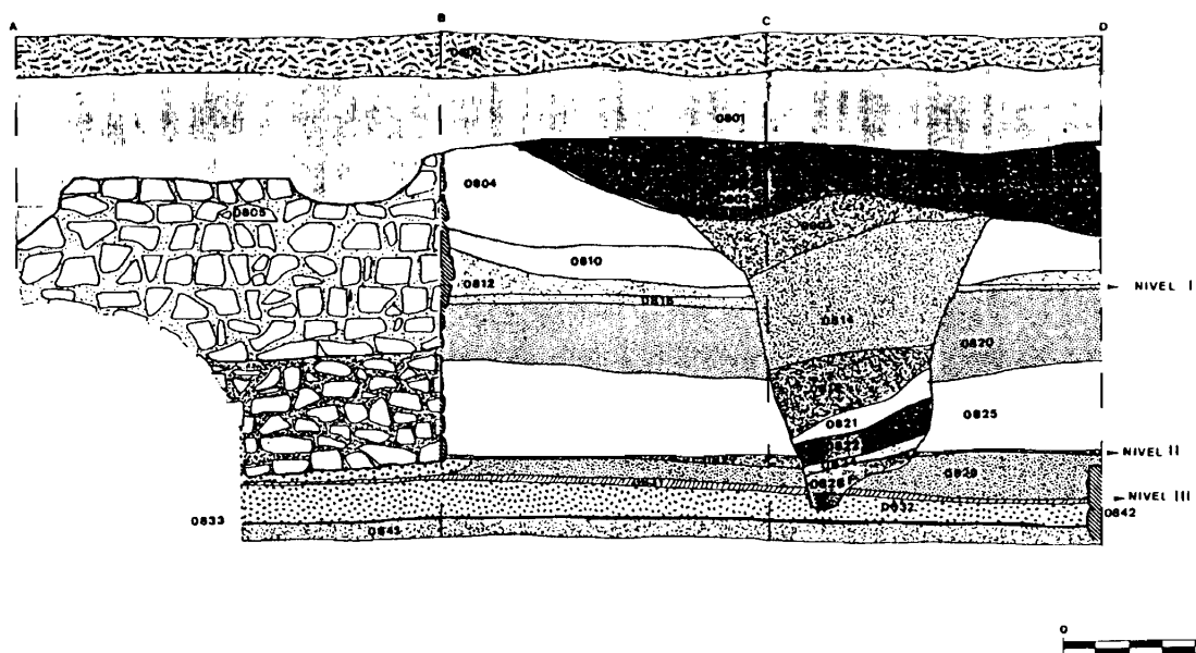
FIGURA 2. Planta y sección del ambiente 1.
