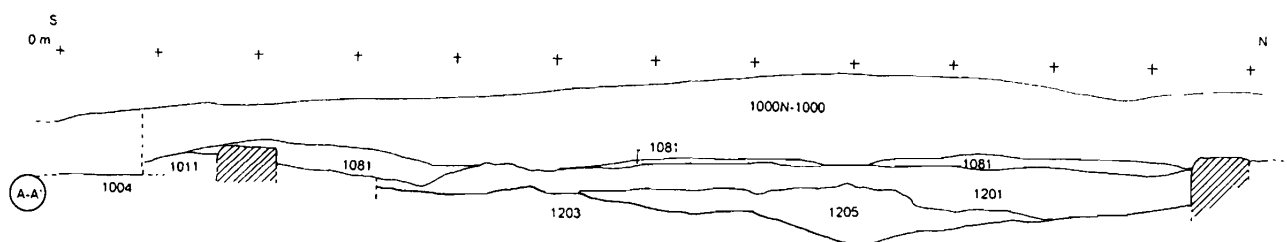
FIGURA 4. Sondeo Natatio. Sección A-A'.
