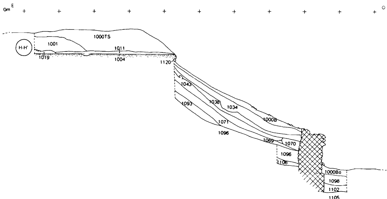
FIGURA 2. Sondeos TS, B y Bo. Sección H-H'.
