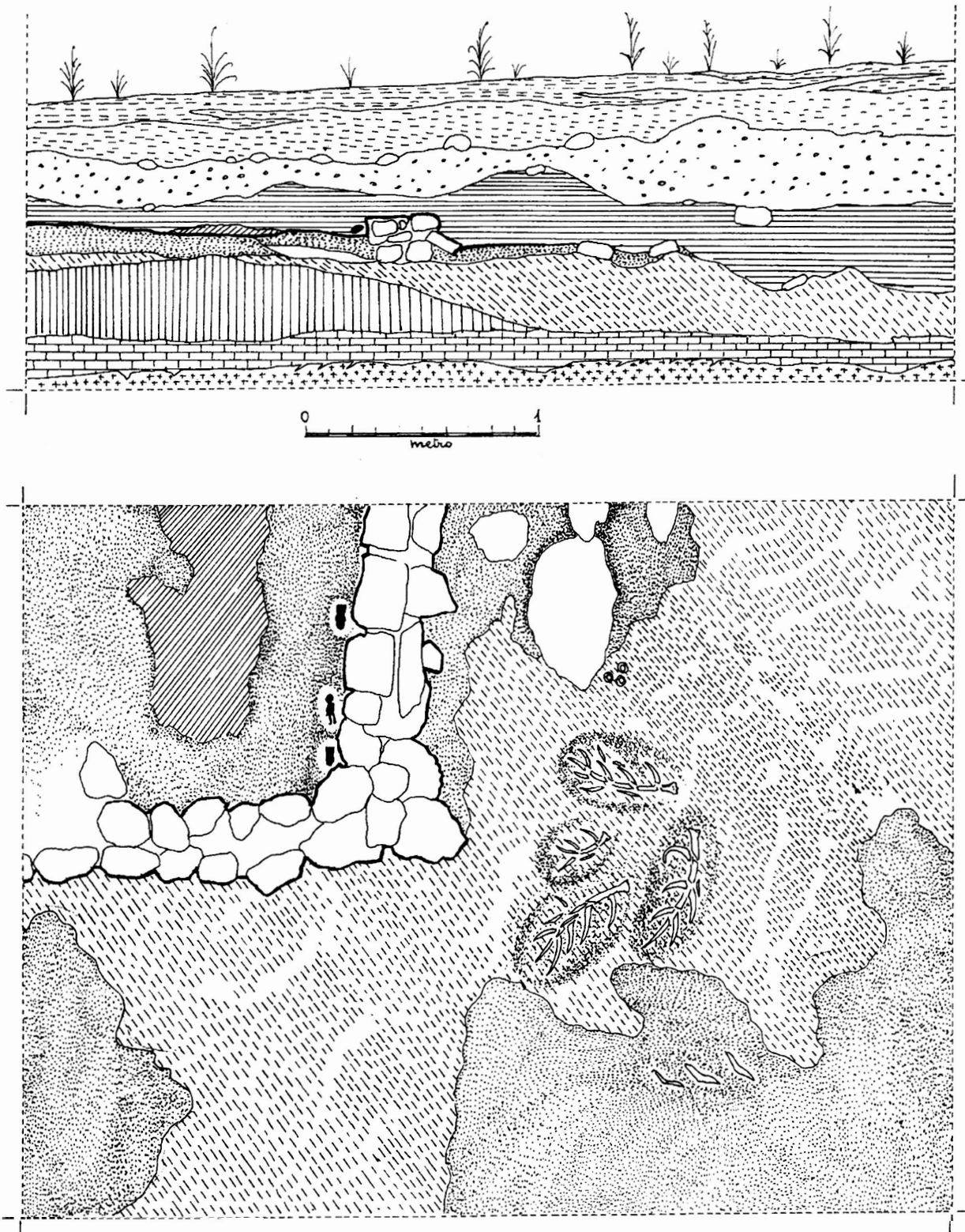
FIGURA 7. Corte P-90. Perfil Norte. En el estrato III vemos la estructura del muro sobre tierra roja. Corte P-90. Planta en el estrato III, con la estructura NW y los exvotos, alineados en su interior. En el exterior, ofrendas de anillos y cuernas de ciervo.
