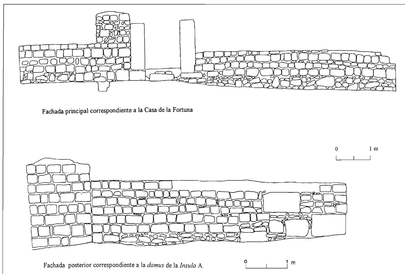
FIGURA 5. Alzados correspondientes a los muros perimetrales de la Domus de la Fortuna y la Domus localizada en la Insula A.
