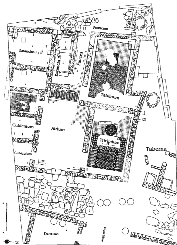
FIGURA 2. Planimetría del conjunto arqueológico de la calle del Duque (Martín et alii, 2001, p. 40, fig 1, y reformado según nuestro estudio).
