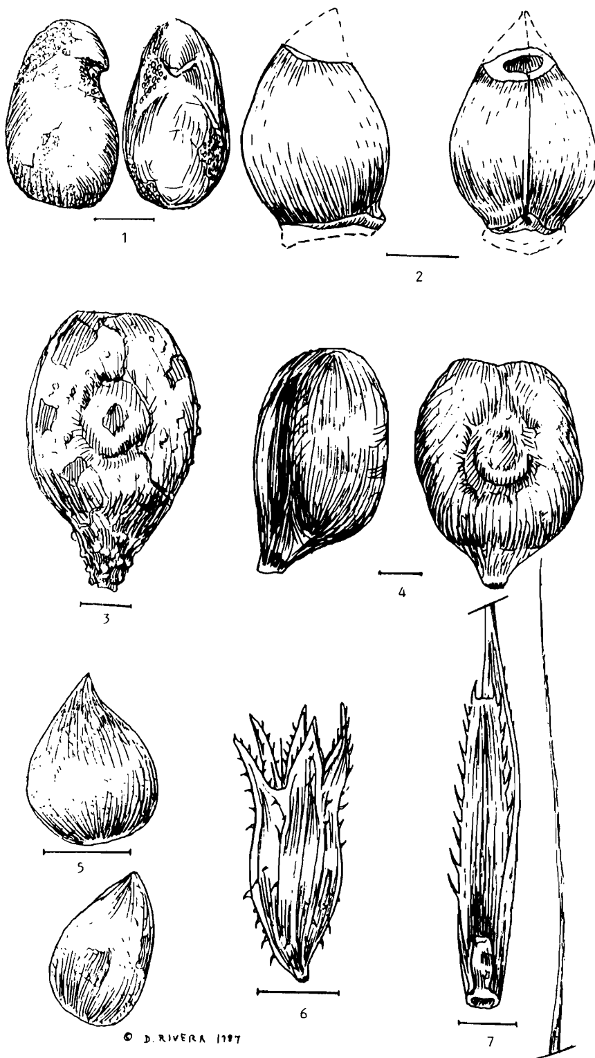
1. Semilla de Capparis spinosa , visión lateral y ventral. 2. Semilla de Lithospermum officinale , utilizada como cuenta de collar, visión lateral y ventral. Los trazos discontinuos muestran las porciones eliminadas por abrasión. 3. Semilla de Vitis vinifera , momificada, visión dorsal. 4. Semilla de Vitis vinifera , carbonizada, visión lateral y dorsal. 5. Semillas de Ficus carica , visión lateral. 6. Cáliz de Satureja gr. cuneifolia , visión lateral. 7. Flor de Trachynia distachya , donde se observa un fragmento de raquis de la espícula, la lema aristada y la pálea bordeada de cilios. (Las líneas que aparecen junto a cada uno de los dibujos representan, en cada caso, la longitud de un milímetro.)
