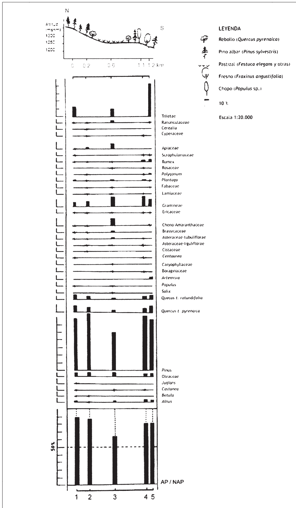
Figura 4. Histograma del transecto de muestras de lluvia polínica, con indicación de altitudes y formaciones vegetales. Figure 4. Transect of pollen rain samples, with indication of plant formations and elevations.
