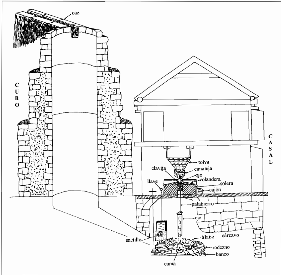
FIGURA 2. Esquema de los elementos del molino de cubo.
