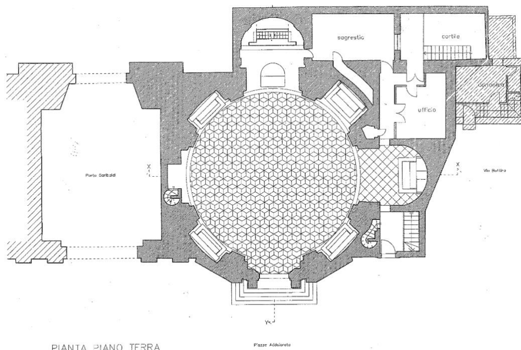
Pianta della Chiesa dell'Addolorata realizzata da Pietro Russo negli anni 1787-1790
