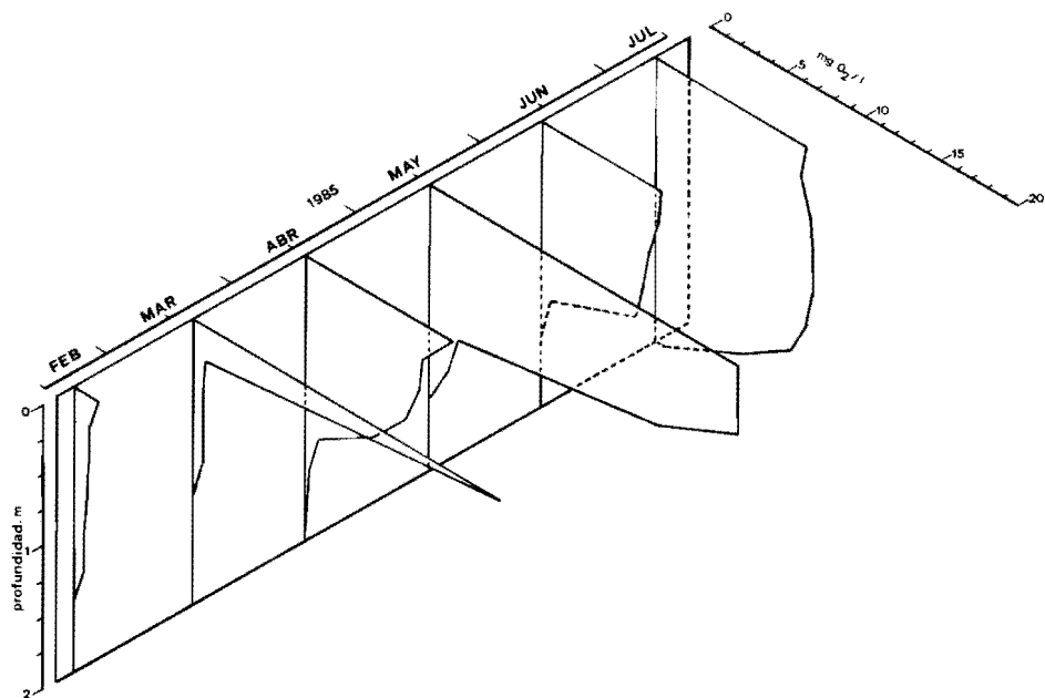
FIGURA 4. Concentración de oxígeno disuelto desde 0 a 2 metros de profundidad durante el primer período de muestreo. Se representan los datos de un solo muestreo por mes.
