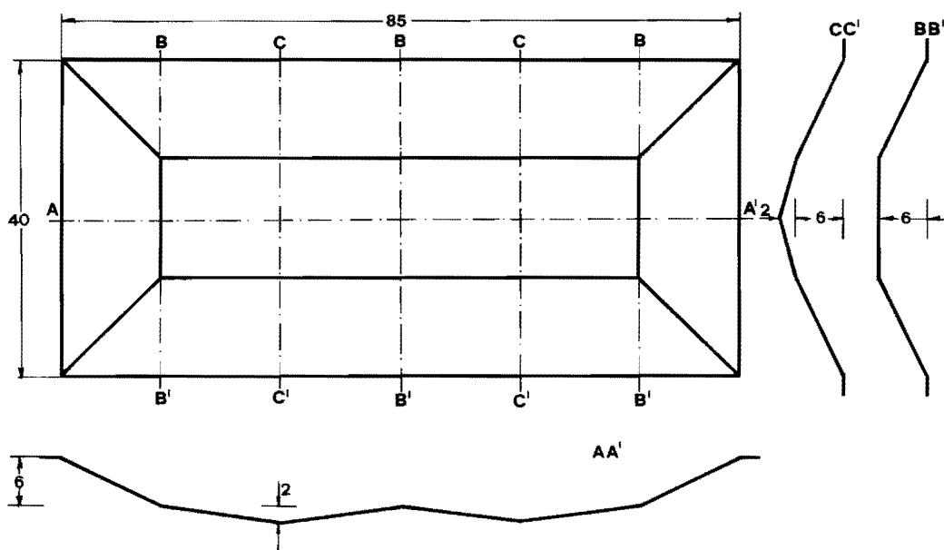
FIGURA 1. Planta y perfiles del estanque de depuración de aguas residuales construido en el Campus de la Universidad de Murcia (dimensiones expresadas en metros).
