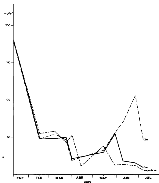
FIGURA 6. Valores de \text{DBO}_5 en superficie, 1 y 2 metros de profundidad en la laguna de autodepuración durante el primer período de muestreo.
