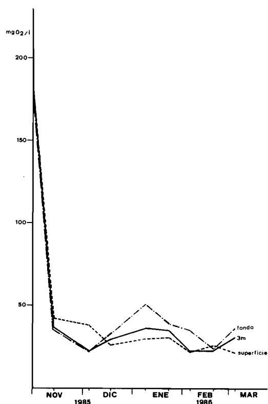
FIGURA 7. Valores de \text{DBO}_5 en superficie, 3 metros y agua del fondo (6,5 a 7 m) en la laguna de autodepuración en el segundo período de muestreo.
