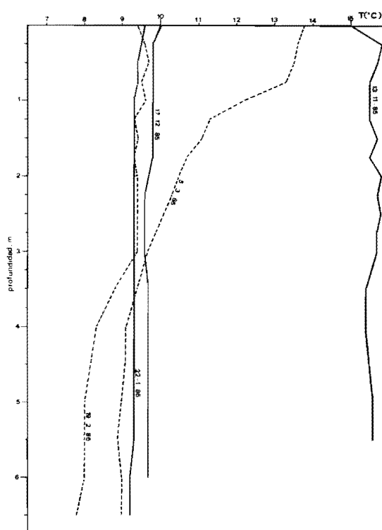
FIGURA 3. Evolución de los perfiles de temperatura en la laguna de autodepuración durante el segundo período de muestreo (noviembre 1985 a mayo 1986). En el mes de marzo se inicia, como en 1985 (ver fig. 2), la formación de la termoclina.
