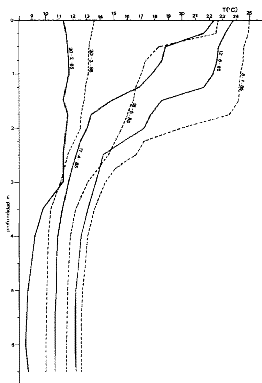
FIGURA 2. Evolución de los perfiles de temperatura en la laguna de autodepuración durante el primer período de muestreo (febrero 1985 a julio 1985). La zona de termoclina inicia su aparición en el mes de marzo y queda estabilizada a partir de julio a los 2 metros de profundidad, aproximadamente.
