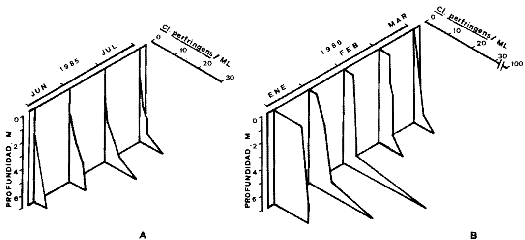
FIGURA 11. Variación de la concentración de Clostridium perfringens respecto de la profundidad y el tiempo en dos fases de distintos períodos de lagunaje. A, aguas altamente depuradas del primer período; B, aguas en proceso de autodepuración del segundo período.
